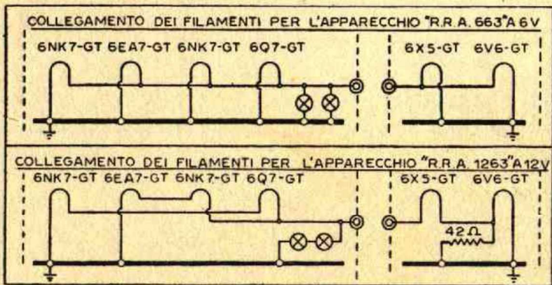
Lo schema elettrico dell'Autovox RRA 663 - RRA 1263.
